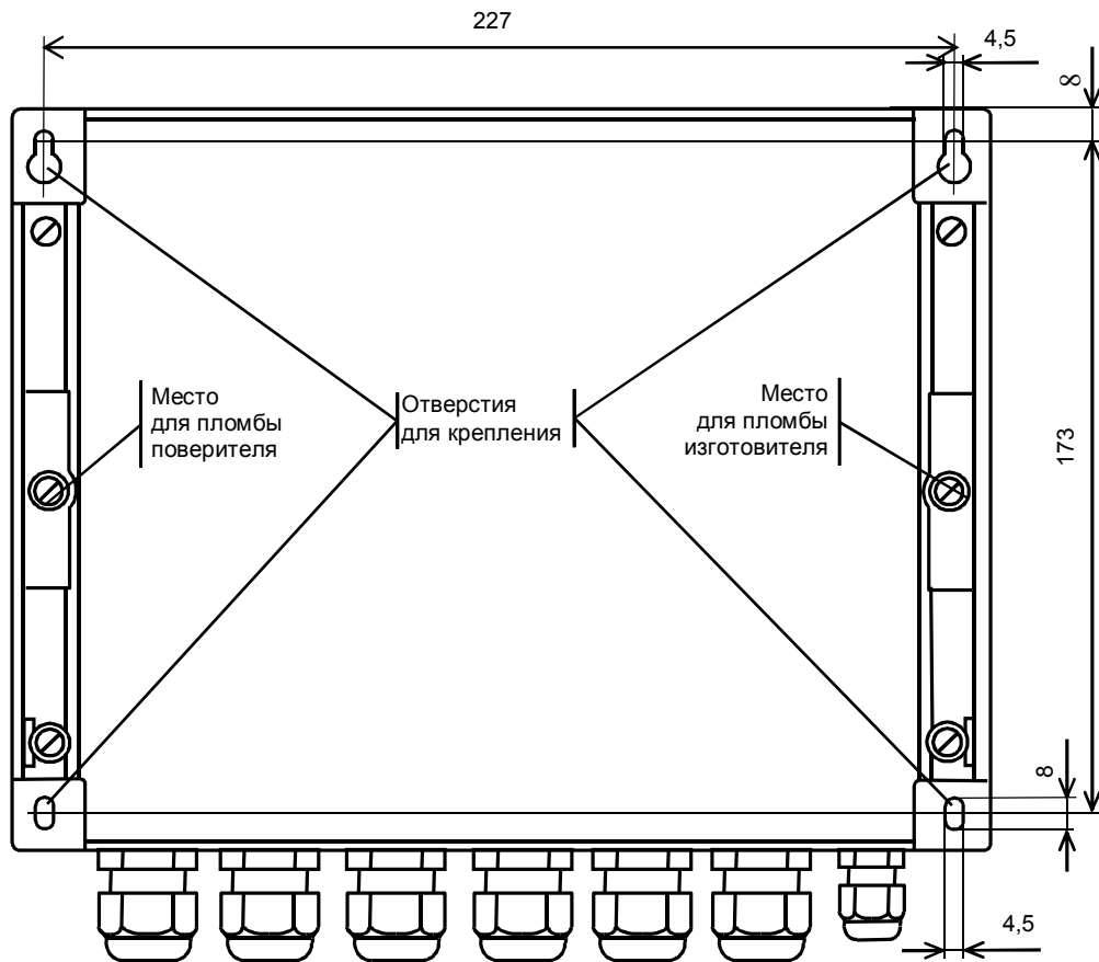
Рисунок 3.3 – Вид сзади
