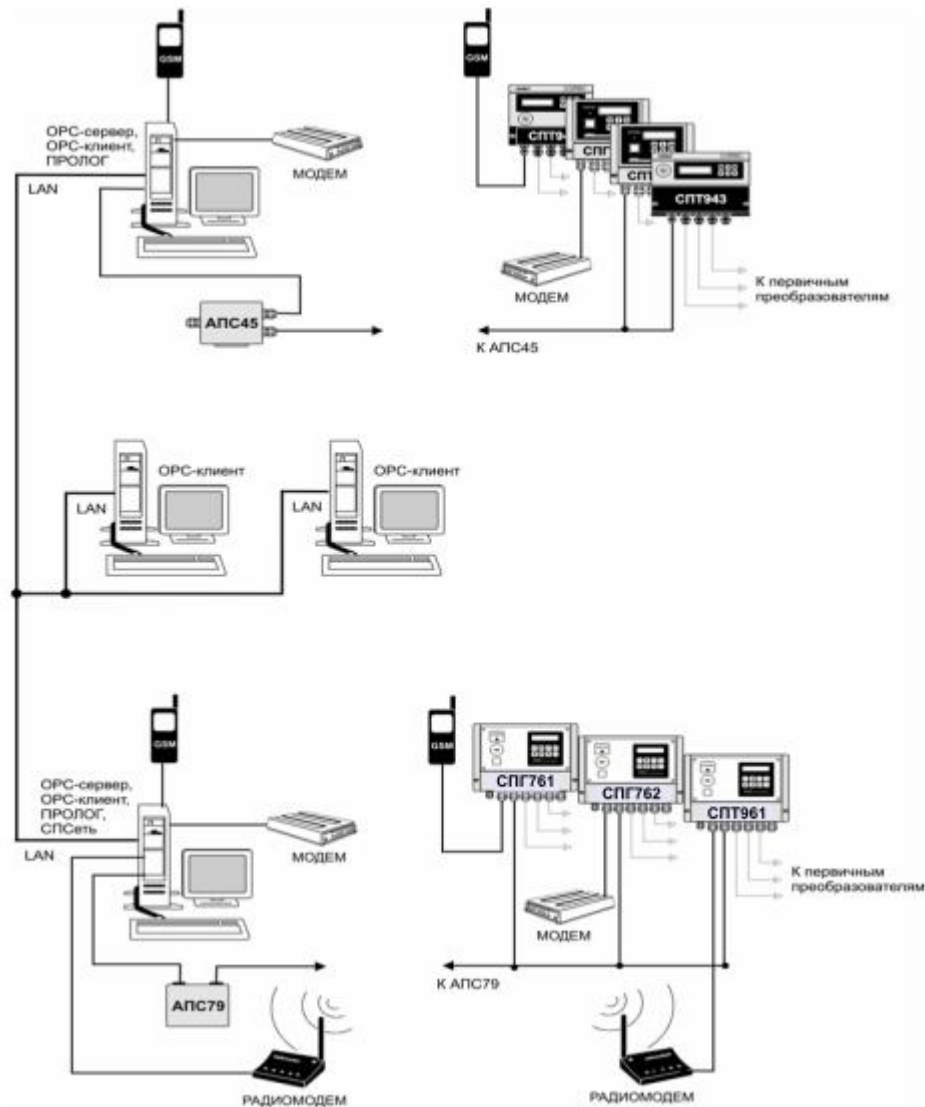
Рисунок 2.2 – Система информационного обеспечения учета энергоресурсов
